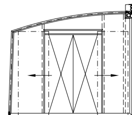
Dvoukřídlé rozsvunuté dveře - fixní čelo
