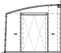
Dvoukřídlé rozsvunuté dveře - fixní čalio
