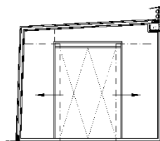
Dvojitákové rozsvinné okno - fixní sklo
